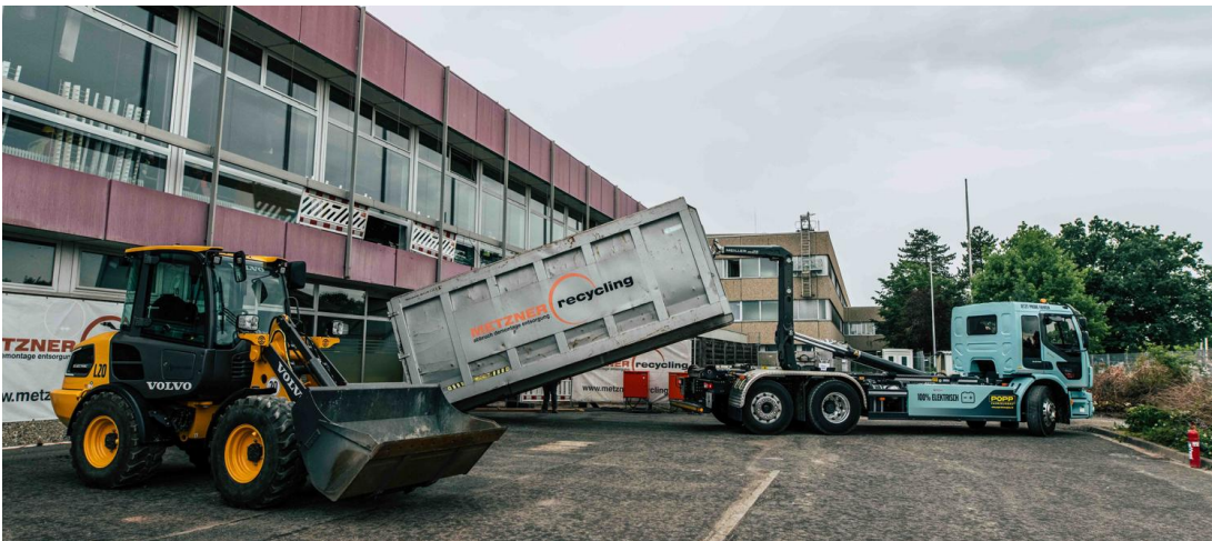
Bild 4: Der Volvo-Radlader L20 Electric übernimmt gemeinsam mit dem Volvo Truck FE 6x2 Electric mit Abrollkipper die Baustellenlogistik.
